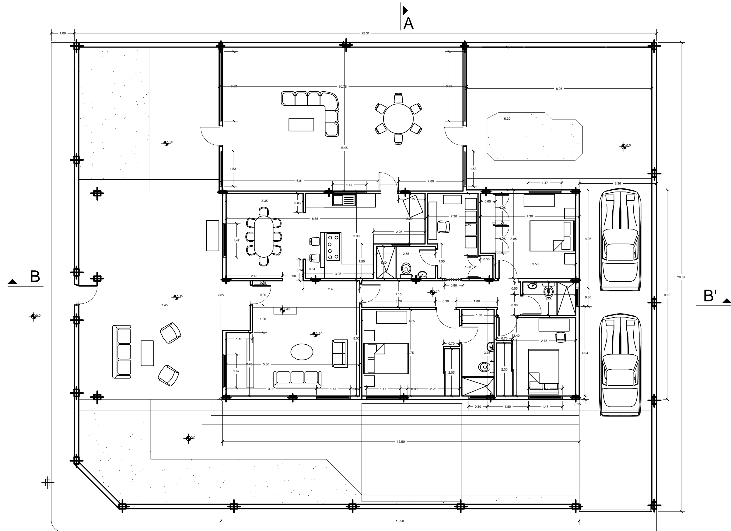
PLANTA DE DISTRIBUCIÓN. ESC. 1:100
